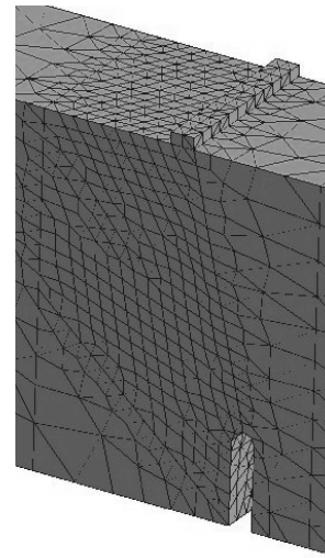
M_4 : 32213 elementos, h \sim 13 [mm]
