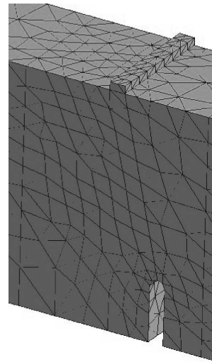
M_1 : 5383 elementos, h \sim 25 [mm]
