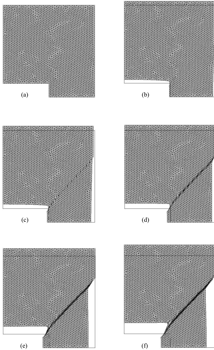
Figura 6.17: Problema de placa con entalla. Secuencia de configuraciones deformadas. Formulaci3n PGPSD-N , Malla M2.
