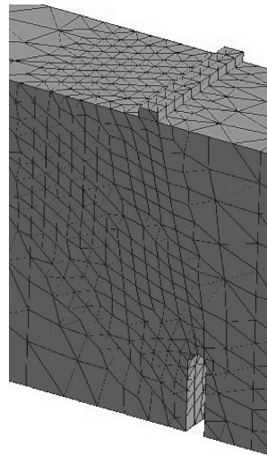
M_3 : 17291 elementos, h \sim 16 [mm]
