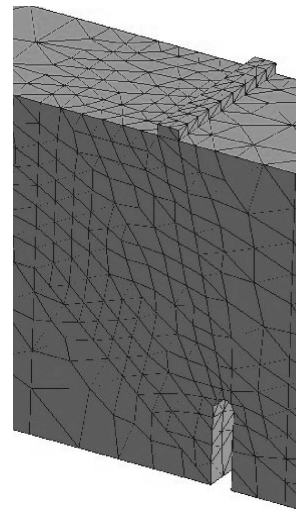
M_2 : 9528 elementos, h \sim 20 [mm]
